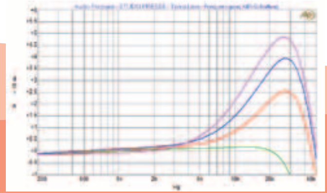
Diagramm 2: Ohne (grün) und mit aktivem Air-Filter bei 14 kHz (rot), 10 kHz (blau) und 7 kHz (magenta)
